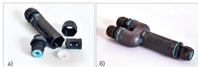
Рис.1. Цилиндрическая система TEETUBE: I-образная (а); Y-образная (б)
