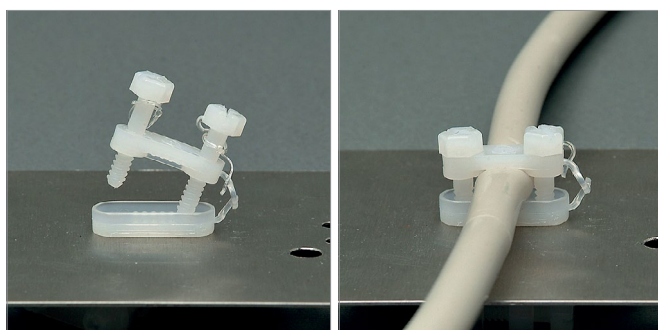
Рис.10. Кабельный зажим TH005
