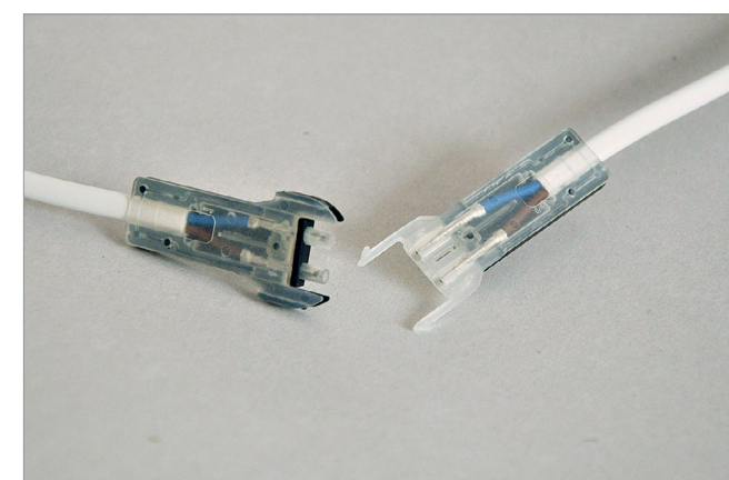
Рис.5. Ультратонкий соединитель TEEPLUG TH420
